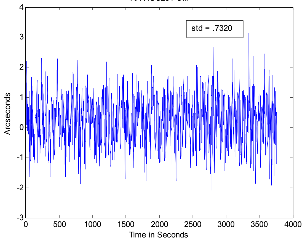
RA NGC281 OIII
