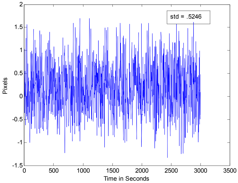
RA NGC6960 SII
