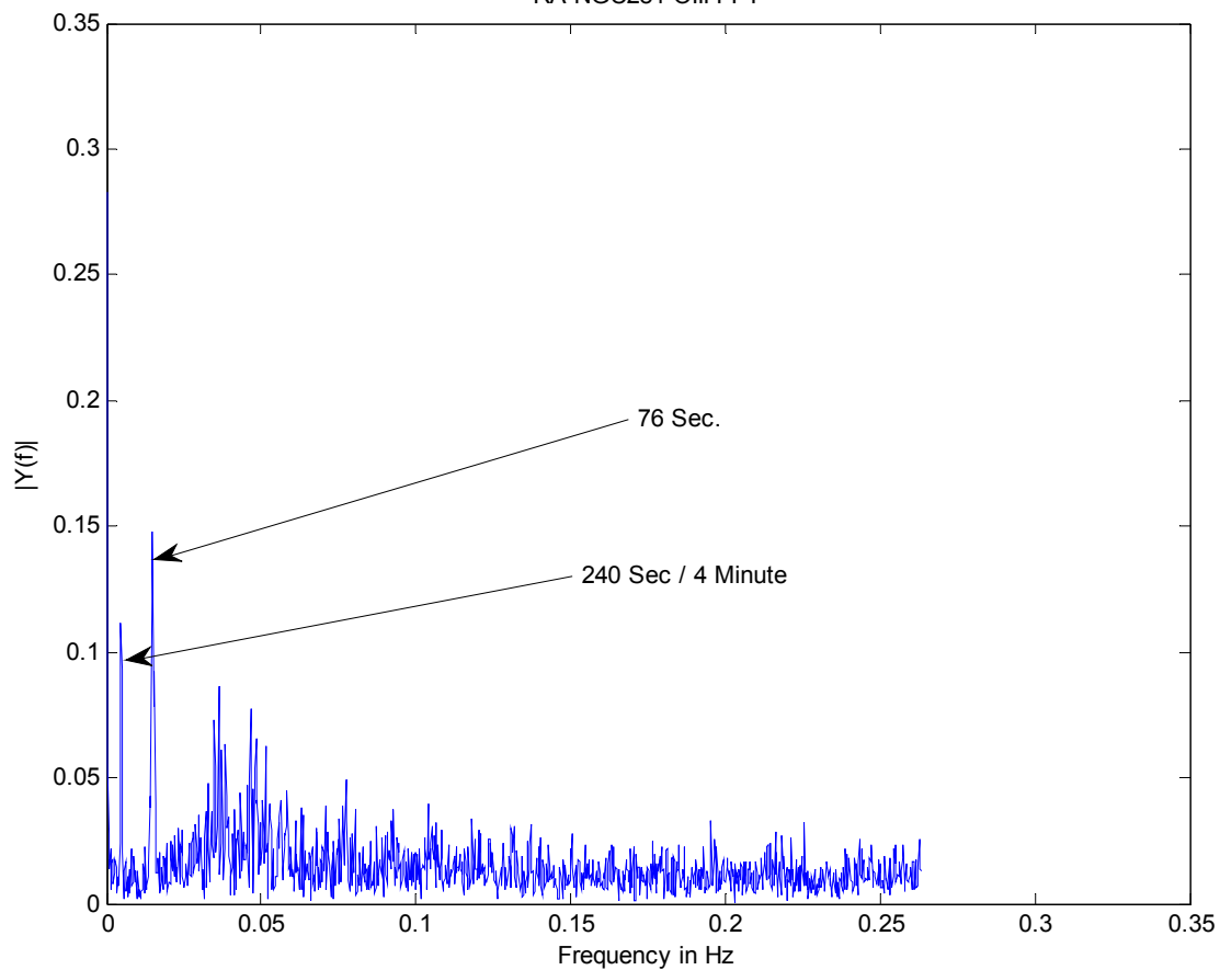
RA NGC281 OIII FFT
